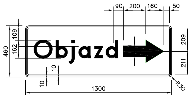
konstrukcja tablicy F-9b
