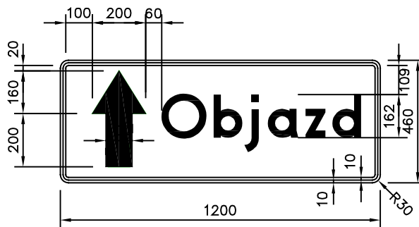
konstrukcja tablicy F-9
