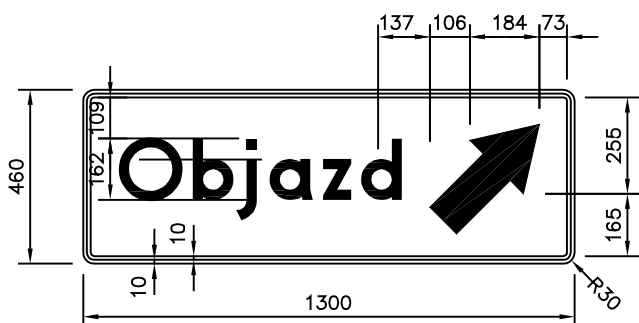
konstrukcja tablicy F-9e
